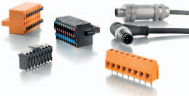
Geräteanschlusstechnik: Leiterplattenklemmen und Steckverbinder Feldverdrahtung: M8-, M12-, M16- und M23-Steckverbinder in IP 67
