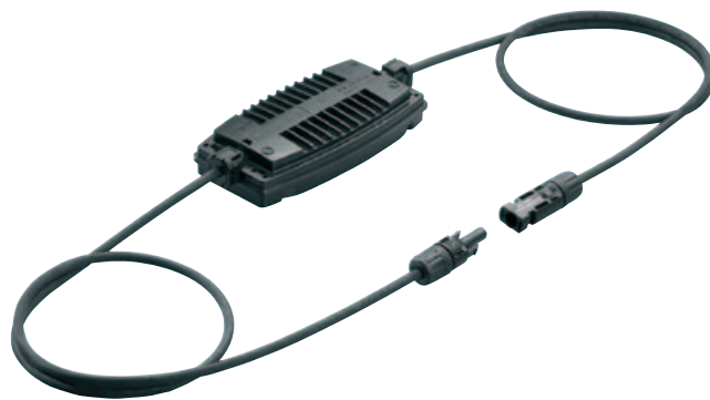
Modulanschluss für effiziente Montage PVM
