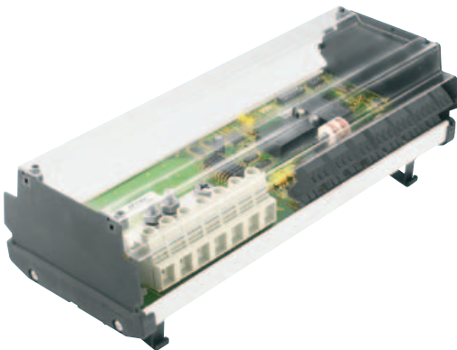
Kontinuierliche Leistungsüberwachung von PV-Anlagen mit Transclinic Xi+ Monitoringsysteme
